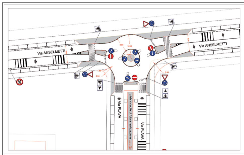
Planimetria 2 - Progetto nuova rotonda al fondo di via Plava
