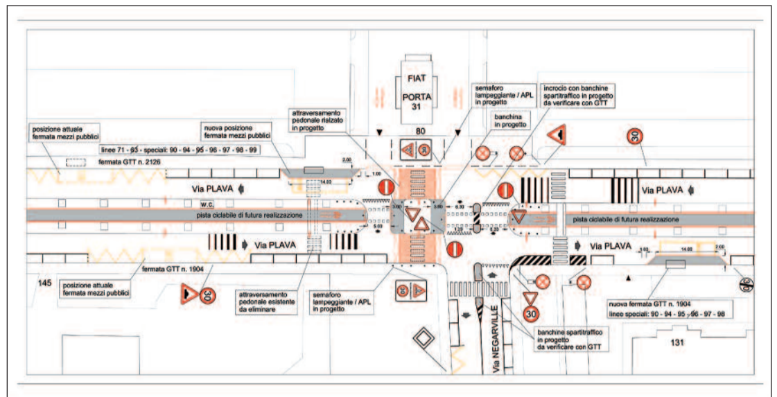
Planimetria 1 - Progetto risistemazione area antistante ingresso 31 (simile soluzione per ingressi 29 e 30)
